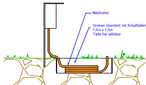
Seitenansicht Bauprovisorium
